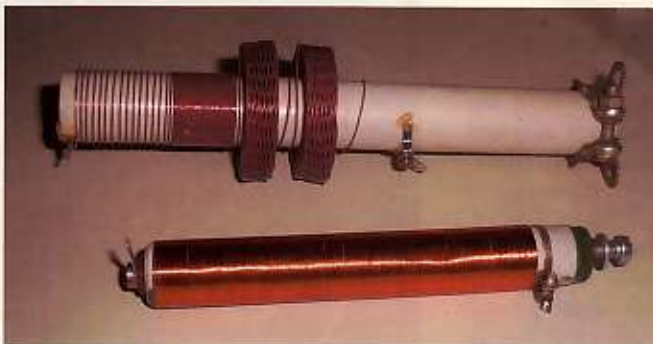
Foto 4: De gewikkelde spoel (onder) en een professionele HF-choke (met de twee ringvormige extra wikkelingen).
